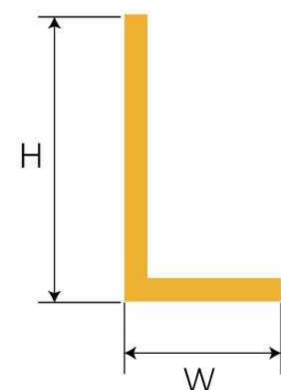
GHL-11x6-74 Unequal Angle
